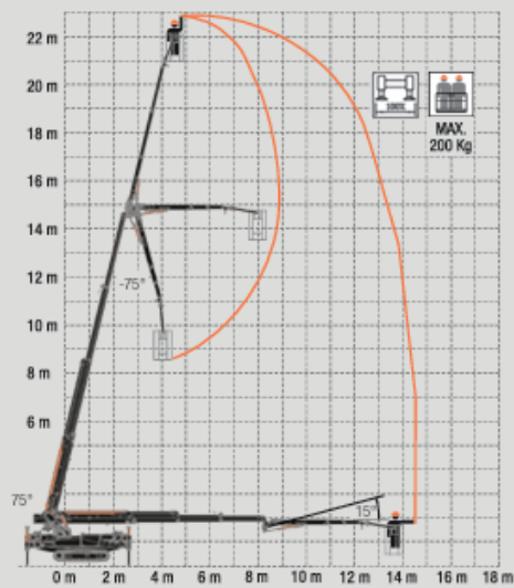
M 400 + Basket
