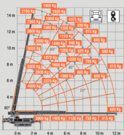
M 400+ Jib
