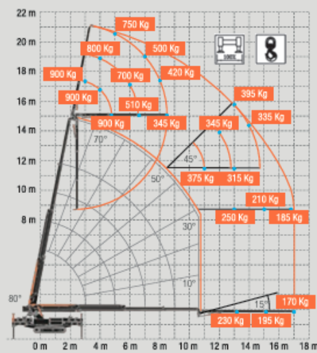
M 400+ Jib
